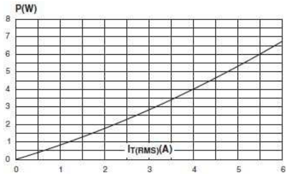
图3 通态特性
