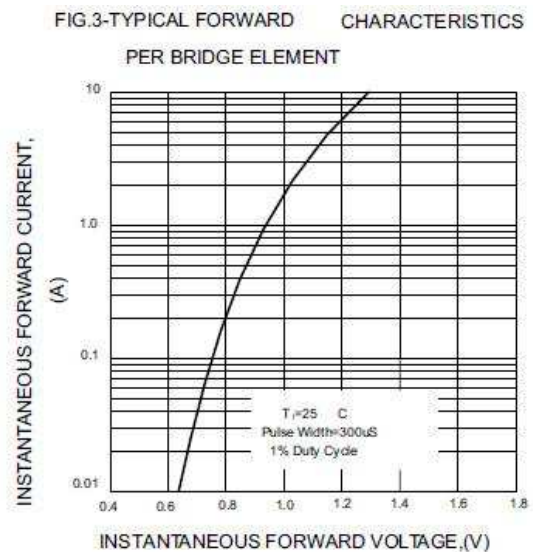
图4. 电性正向特性曲线
