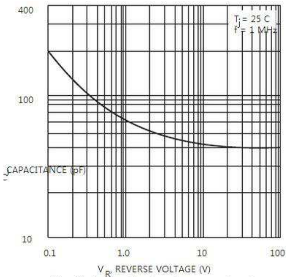
图3. 结电容随反向电压变化曲线
