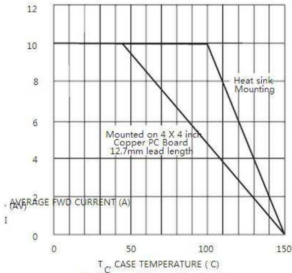
图1. 正向电流随温度变化曲线
