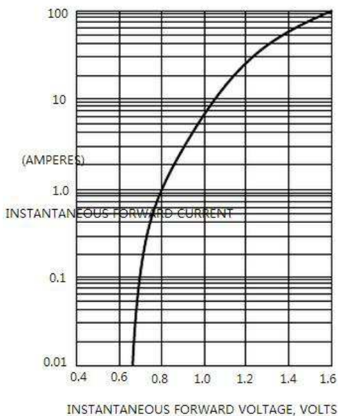
图4. 电性正向特性曲线
