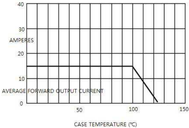
图1. 正向电流随温度变化曲线
